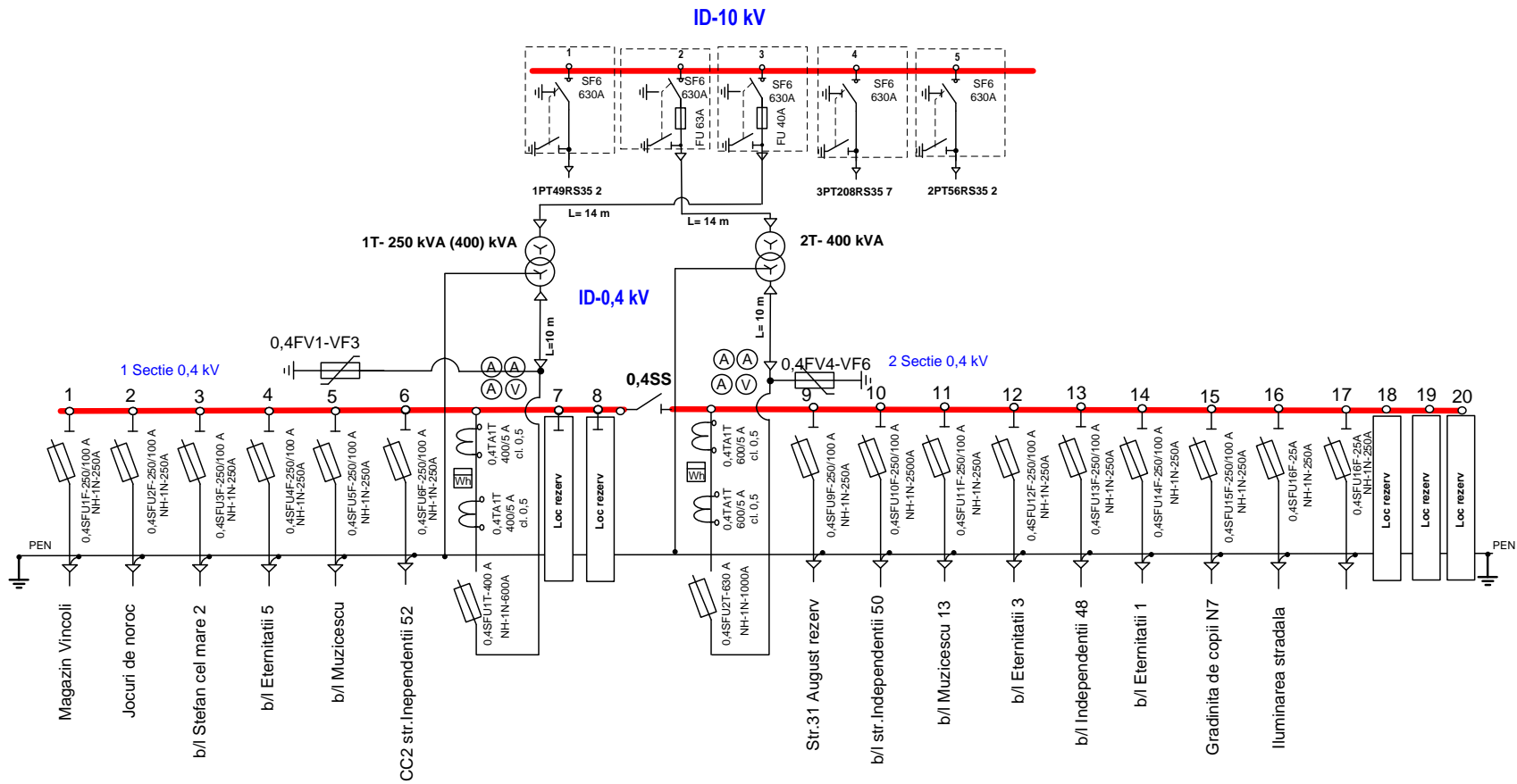
Schema monofilară a utilajului la PT5RŞ35 2 or.Rișcani
